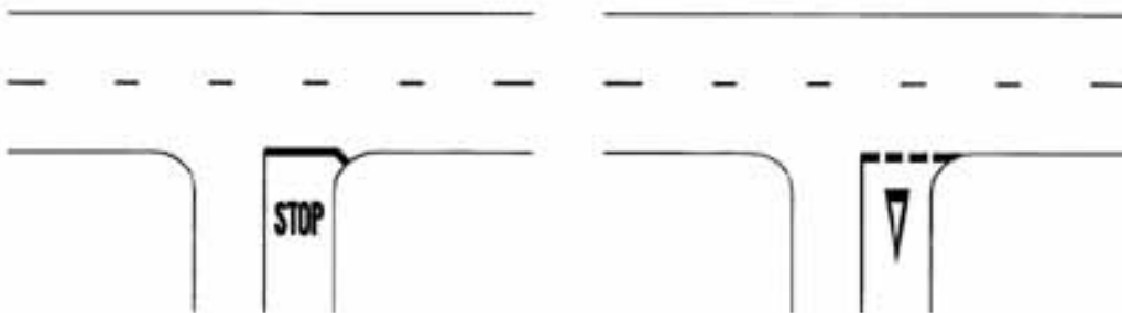
Megállást és elsőbbségadást jelző útburkolati jelek
