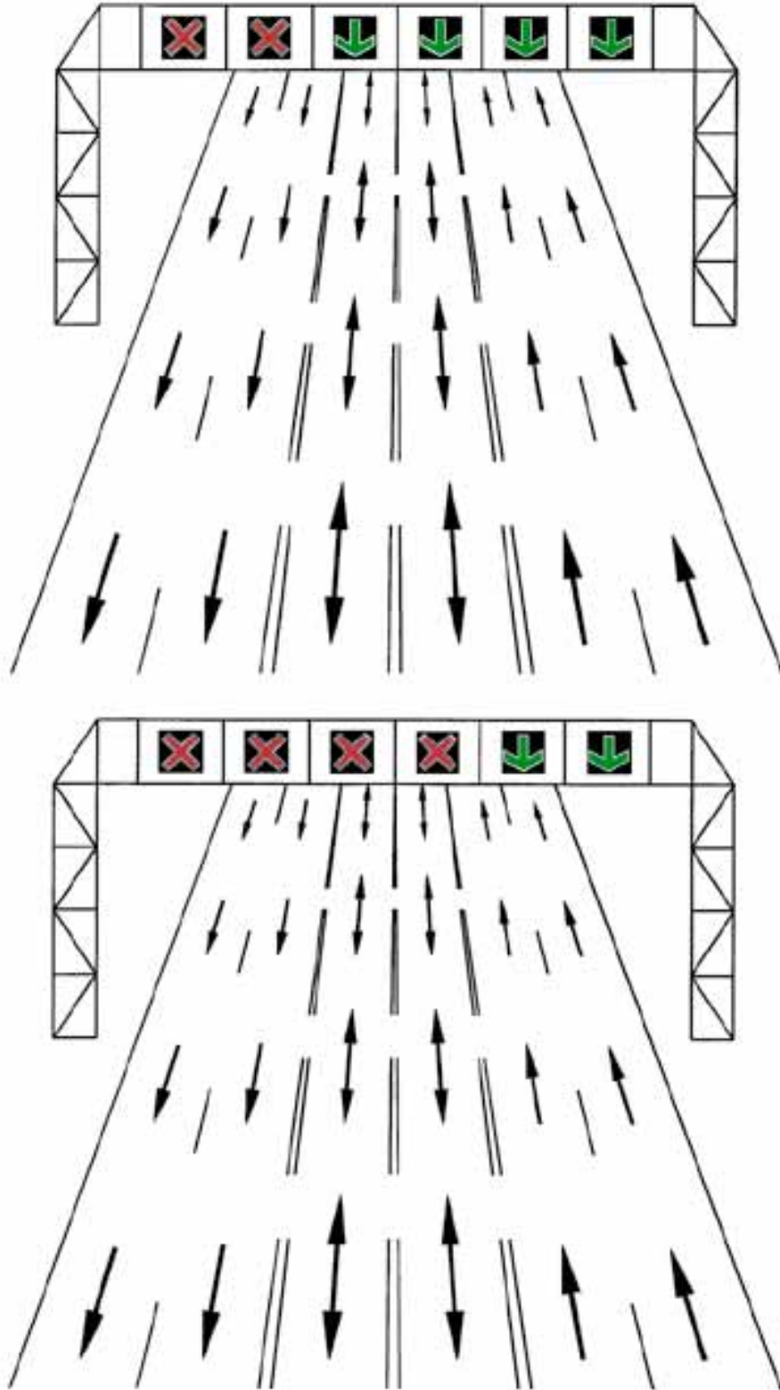
A járműforgalom irányítására szolgáló fényjelző készülékek változóirányú sávokon
